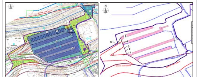
Чертеж планировки и межевания территории План красных линий. Разбивочный чертеж
